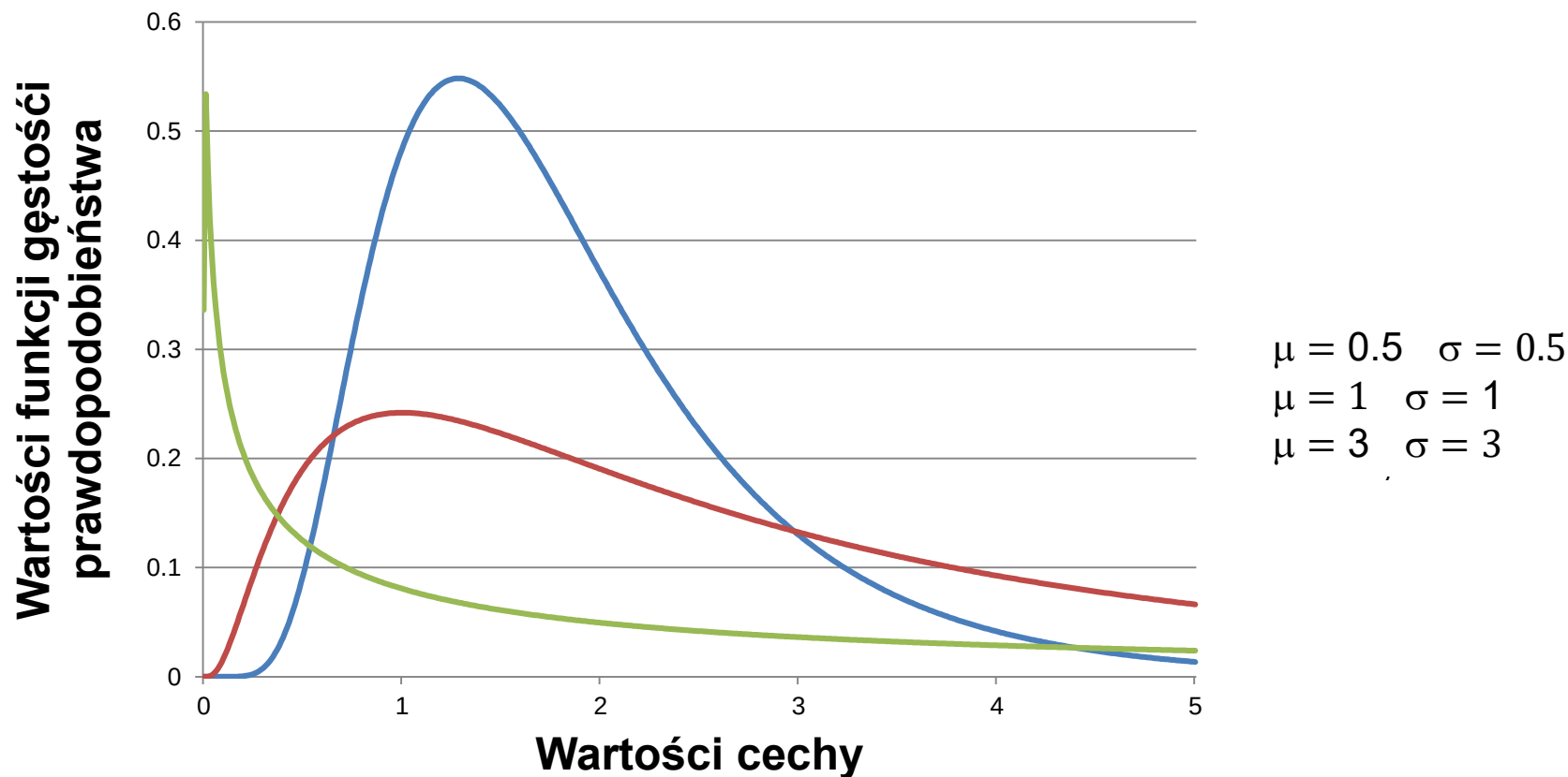
Funkcja gęstości rozkładu log-normalnego
