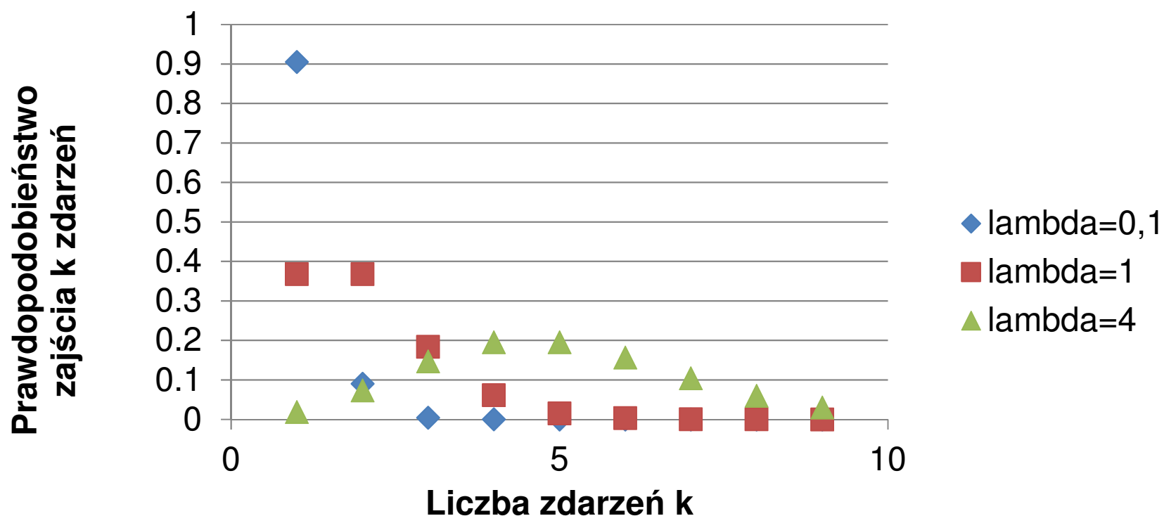
Funkcja gęstości rozkładu Poissona przy \lambda=0.1; 1; 4
